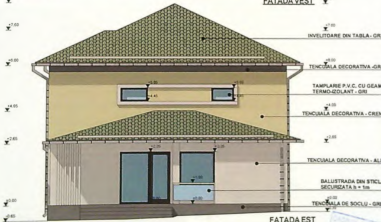
FATADA EST
